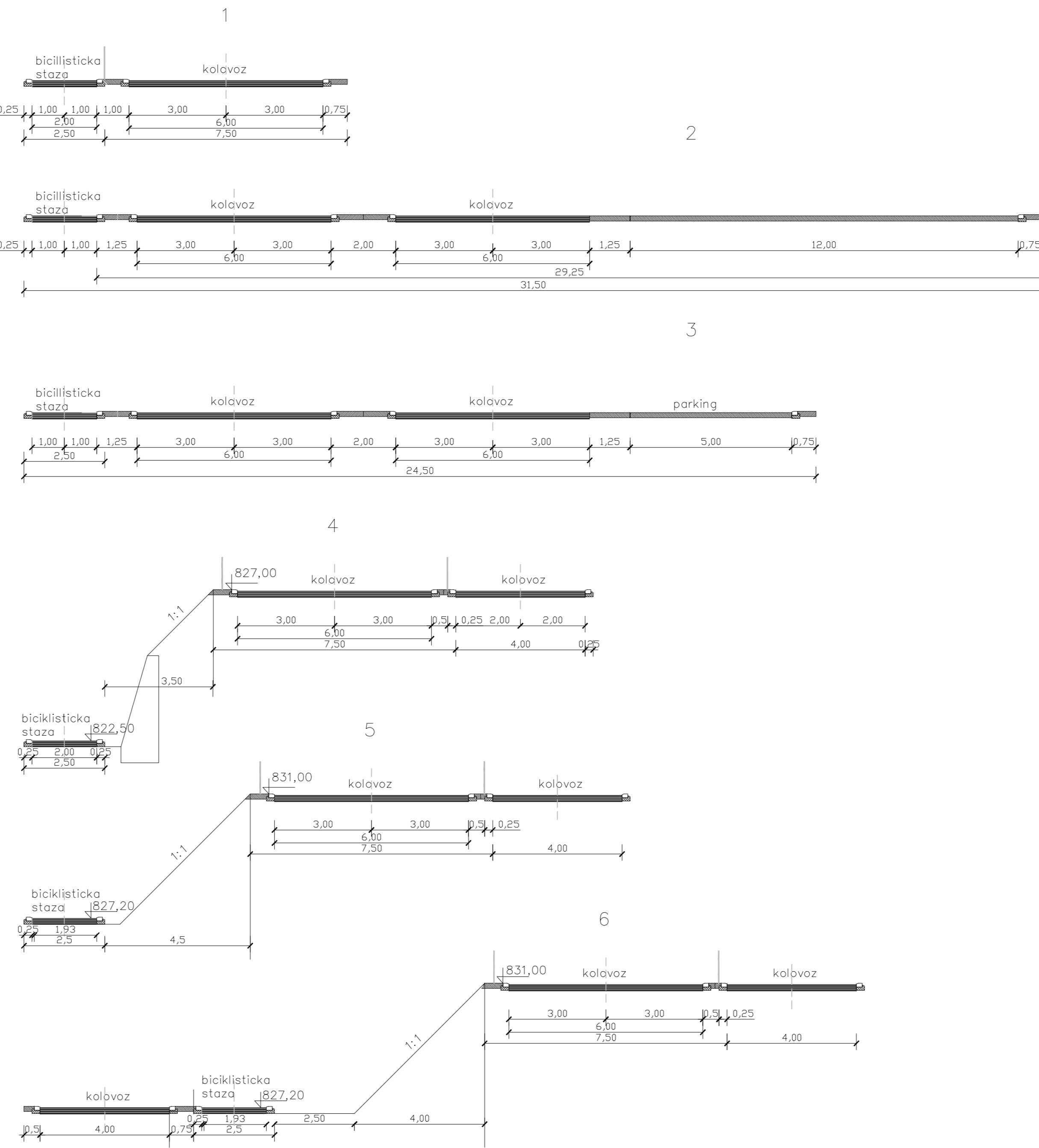
NORMALNI PROFILI R=1:100
